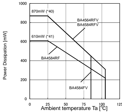
(d)BA4564R/BA4584/BA4584R family
