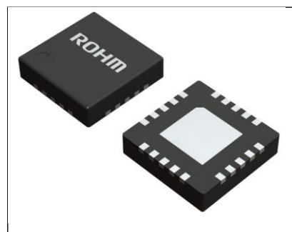
VQFN020V4040
