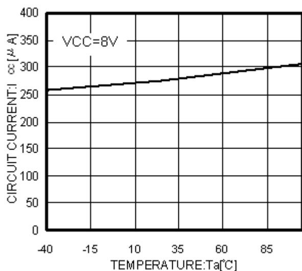
Fig.12 T_a - I_{cc}
