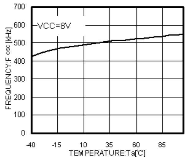
Fig.9 Ta-FOSC
