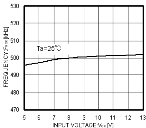
Fig.13 V_{CC} - F_{OSC}
