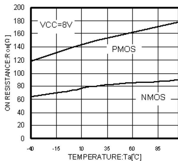
Fig.10 Ta-RONN, RONP
