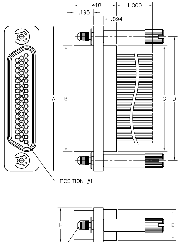
RECEPTACLE
