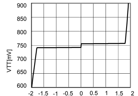
Fig.12 ITT-VTT(DDR3)
