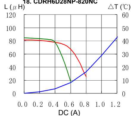
18. CDRH6D28NP-820NC
