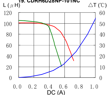
19. CDRH6D28NP-101NC
