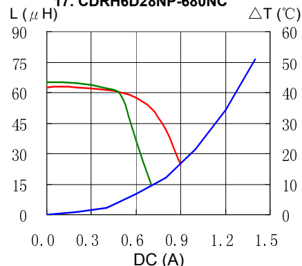
17. CDRH6D28NP-680NC
