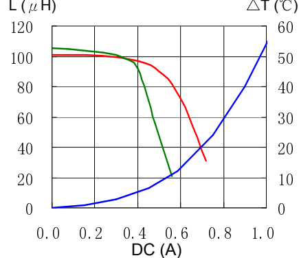
19. CDRH6D28NP-101NC
