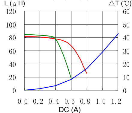
18. CDRH6D28NP-820NC
