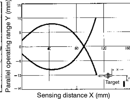
E32-D32 with E3X-A11 amplifier
