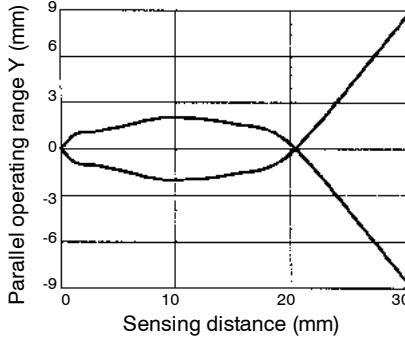
E32-D32 with E3JU-XR amplifier
