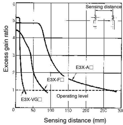
E32-T14L with E3X-A, E3X-F and E3X-VG amplifiers
