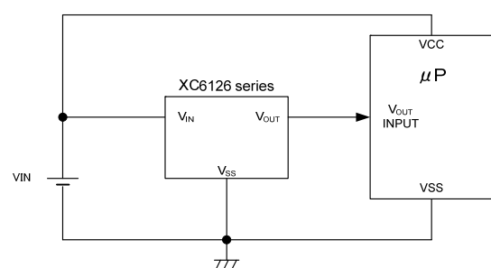
CMOS output
