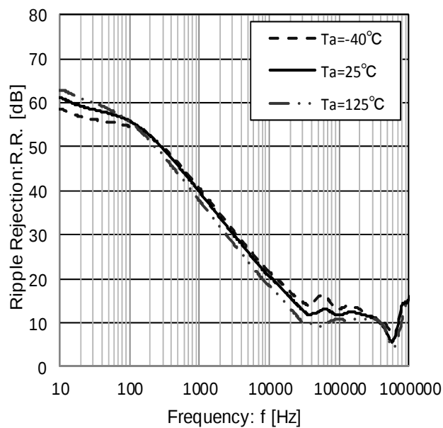
Figure 28. Ripple Rejection (I O =100mA)
