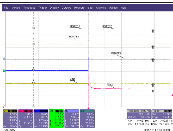
Figure 21. Hot Plug VIN2 VIN1 > VIN2
