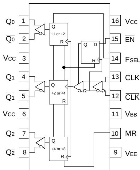
16-Pin SOIC (Z16-2)
