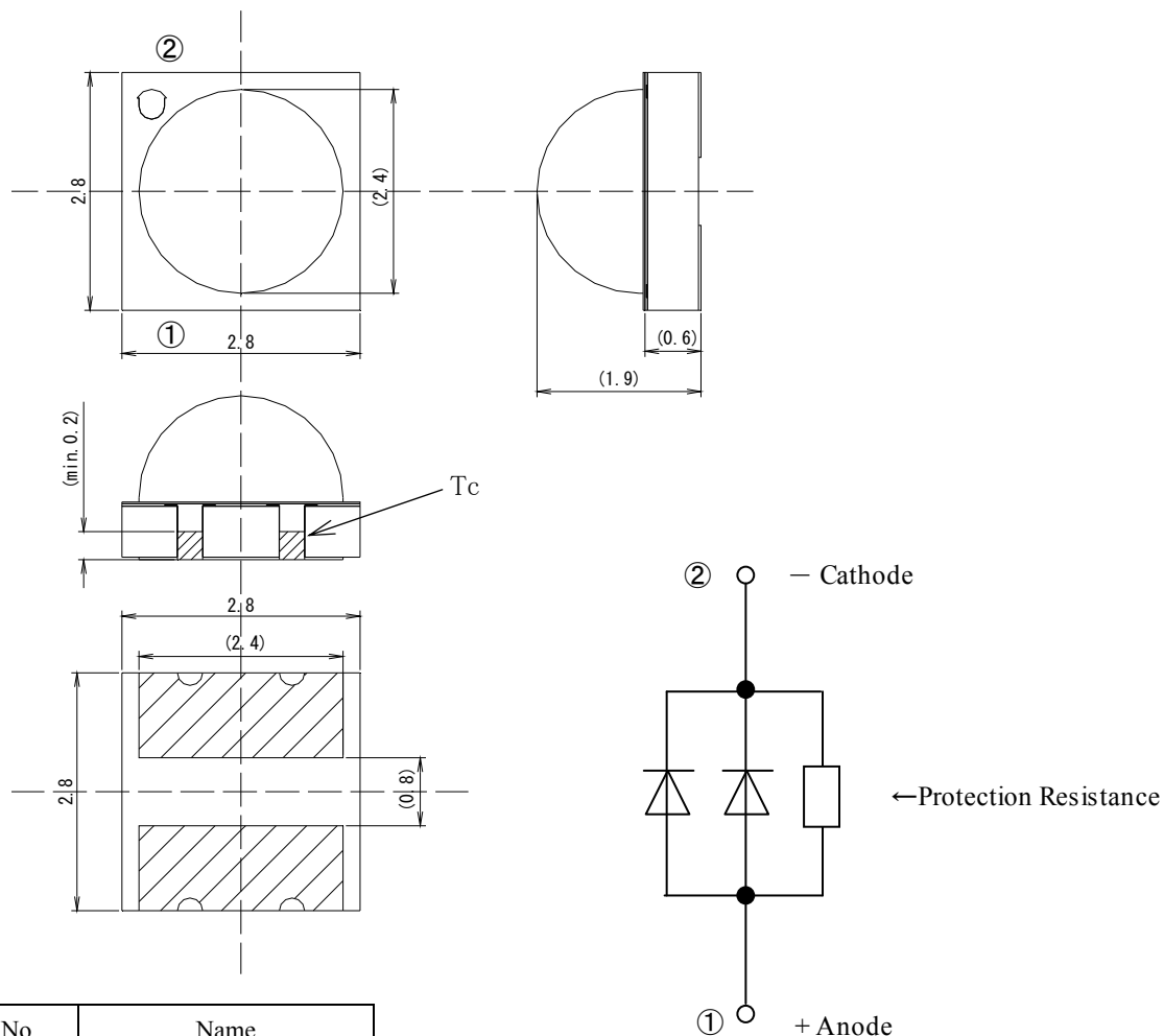
内部等価回路図 Equivalent circuit
