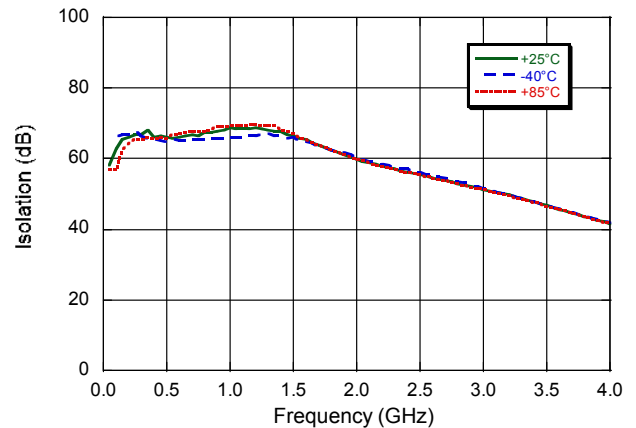
Isolation_RFC - RF1
