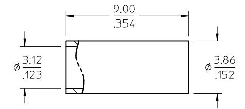
FERRULE
