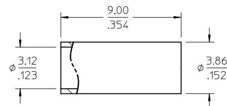
FERRULE
