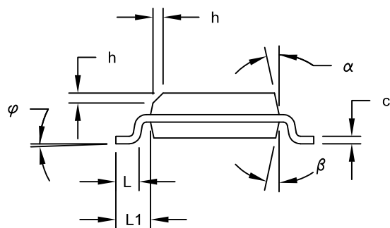
VIEW A-A
