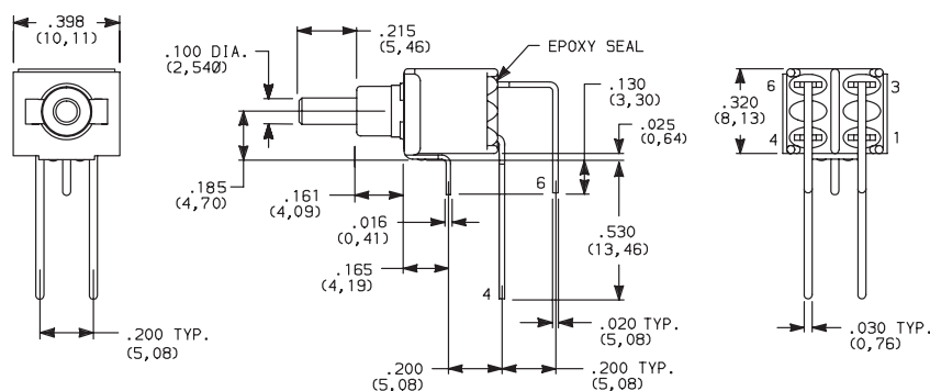
EP21SD1AVBE DPST
