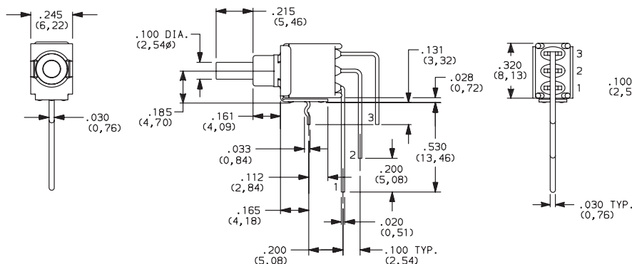
EP12SD1AV3BE SPST
