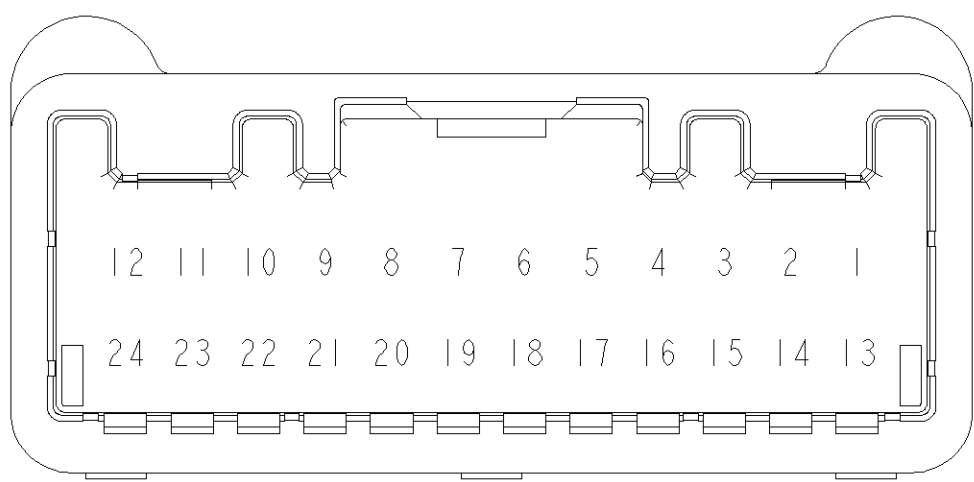
FIG. 1 CONTACT POSITION コンタクト回路構成
