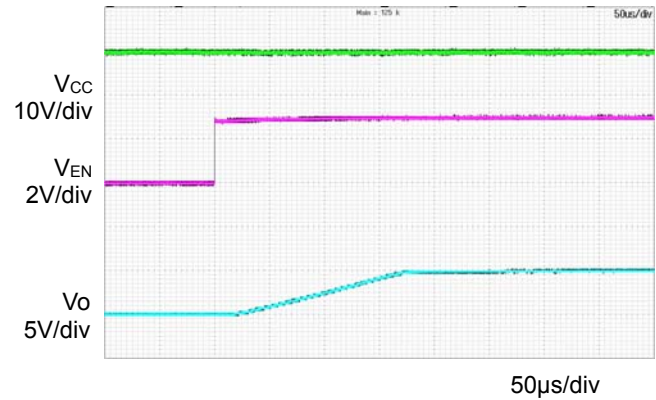
Figure 6. Input sequence (Ta=-40°C) (EN = 0V→3V)
