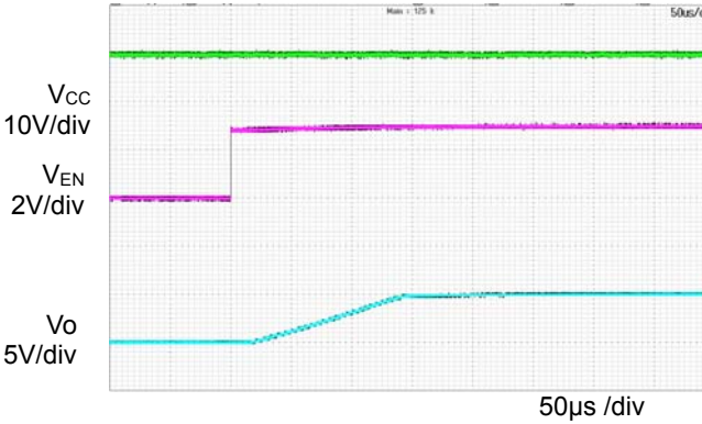
Figure 5. Input sequence (Ta=25°C) (EN = 0V→3V)
