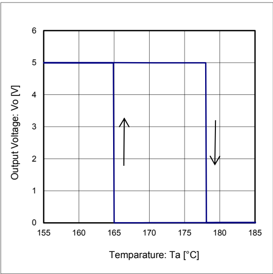
Figure 22. TSD (Io = 0mA)
