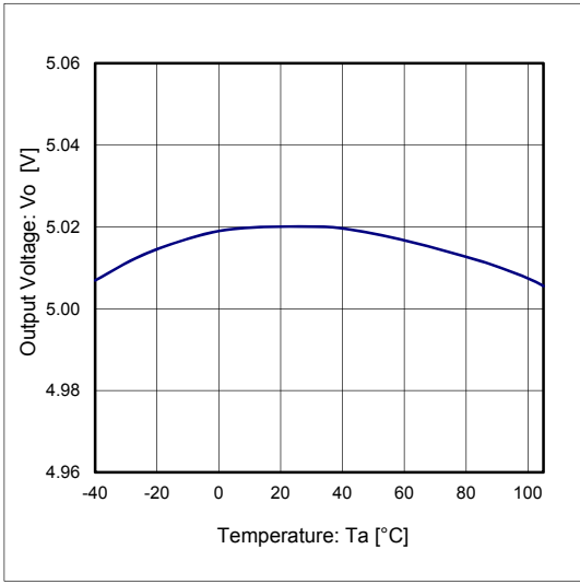
Figure 15. Ta - Vo (Io = 0mA)
