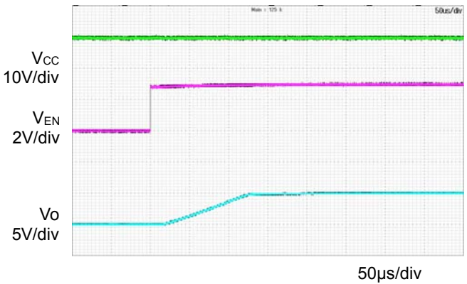
Figure 7. Input sequence (Ta=105°C) (EN = 0V→3V)
