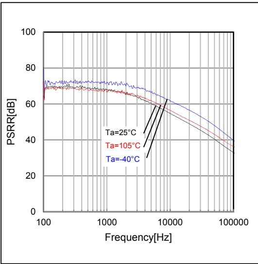
Figure 24. PSRR (Input Voltage Ripple = 1Vrms, Io = 50mA)
