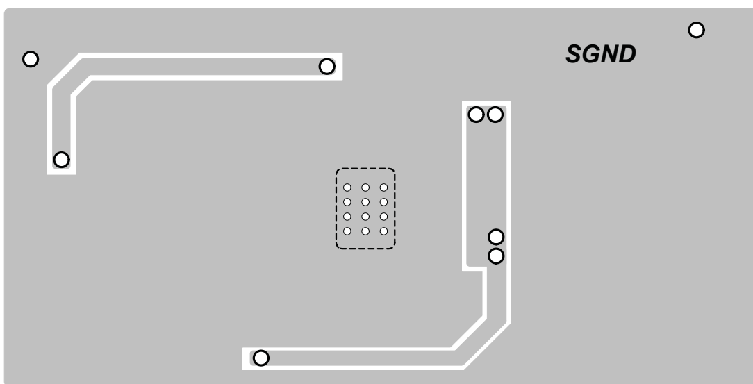
Bottom Layer
