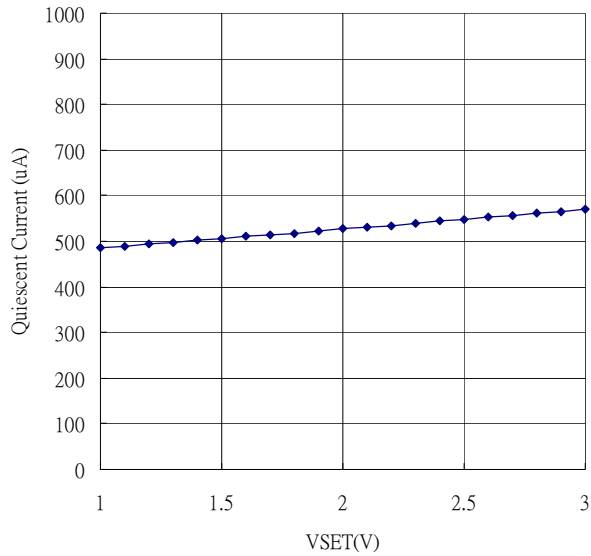
VSET V.S. QUIESCENT CURRENT
