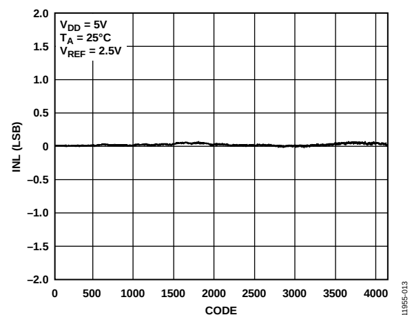
Figure 13. AD5681R INL
