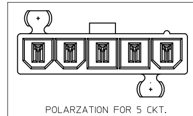
POLARIZATION FOR 5 CKT.
