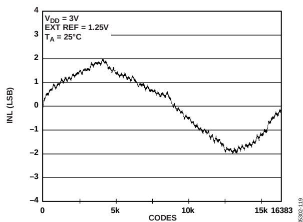
Figure 20. INL AD5648-1
