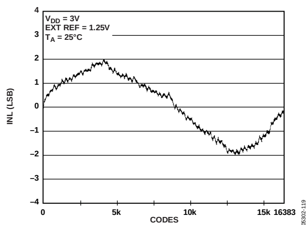
Figure 20. INL AD5648-1
