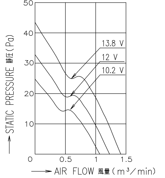
風量-静圧特性例
