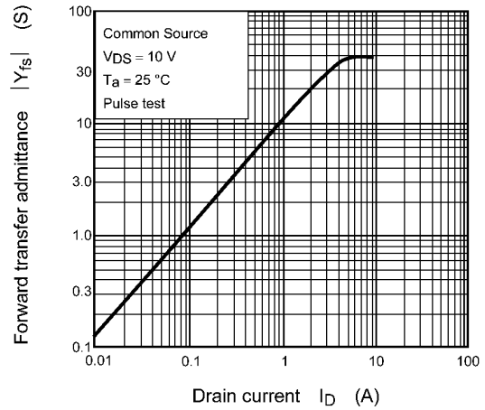
Fig. 7.8 |Y_{fs}| - I_D
