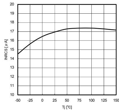
Fig.20 Tj-NRSC
