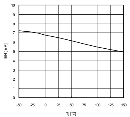
Fig.21 Tj-IEN
