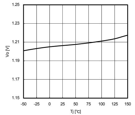
Fig.15 Tj-Vo ( I_o=0\text{mA} )
