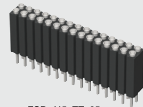
ESD-115-TT-05
