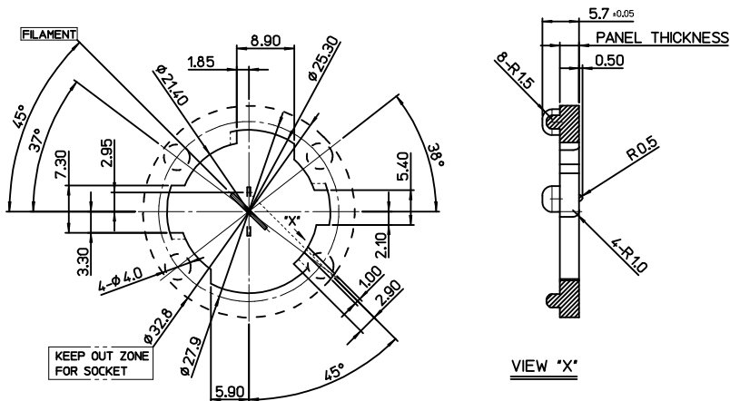
LUG PATTERN "A"
