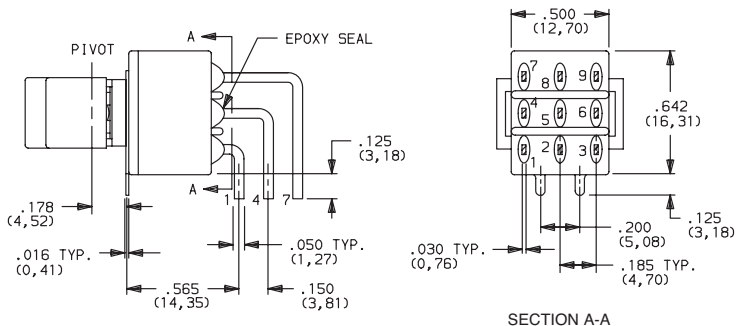
E301J1ABE2 Horizontal Actuation 3PDT
