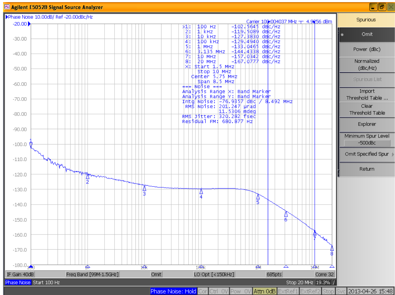
Phase Noise Plot: 100MHz, 1.5MHz – 10MHz 320fs
