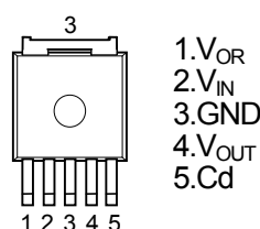
NJM2806DL3
