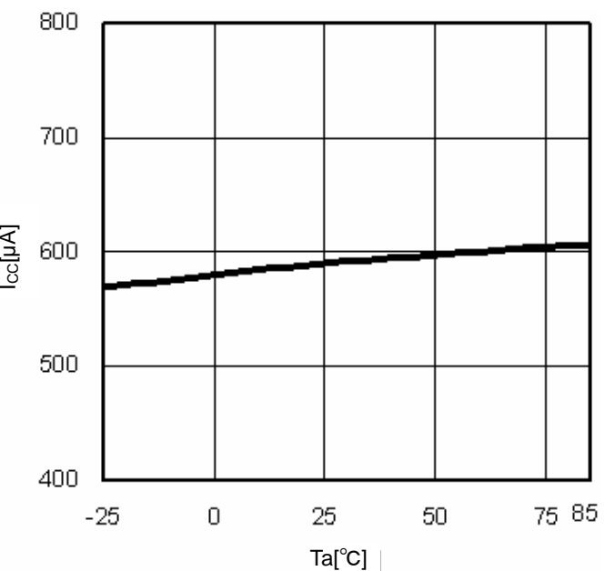
Fig.9 Ta-I CC
