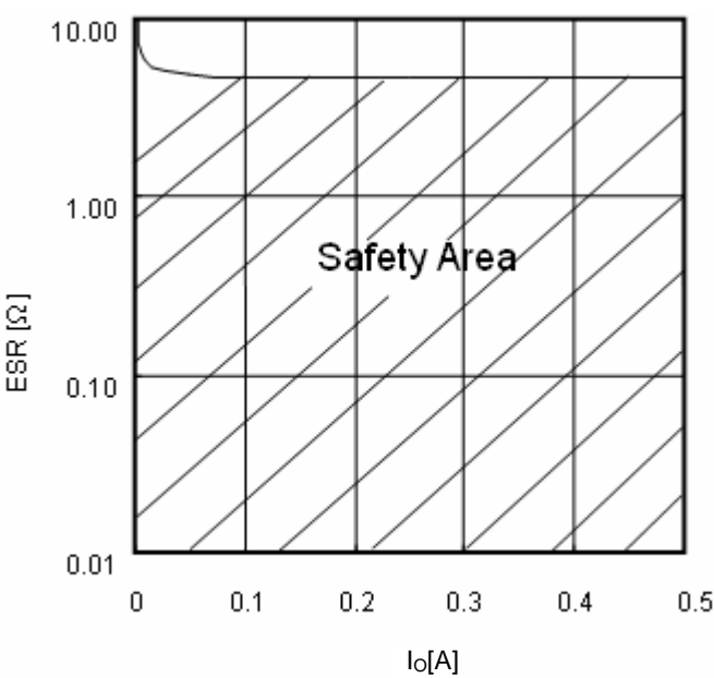
Fig.18 ESR condenser
