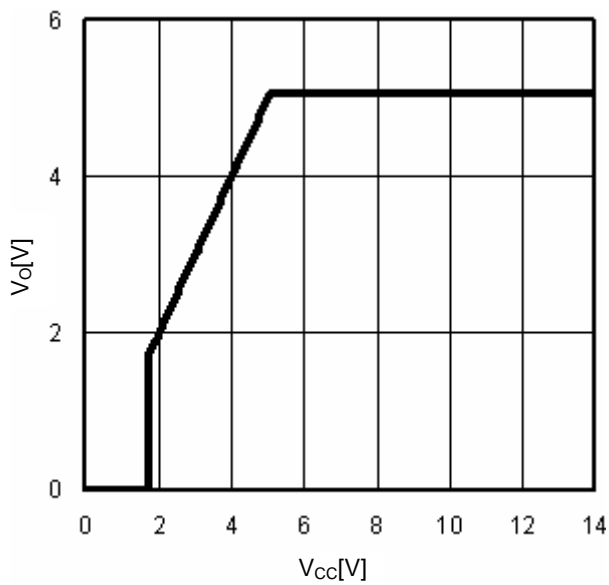
Fig.14 V_{CC}-V_O ( I_O=0\text{mA} )
