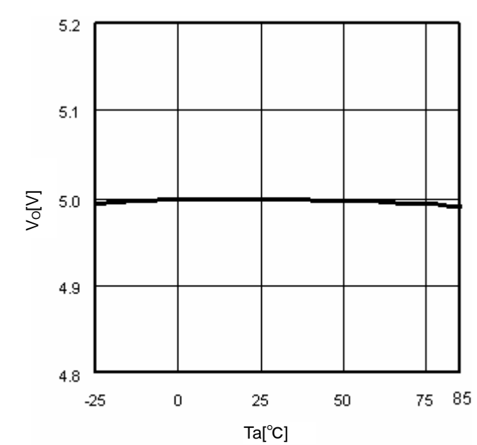
Fig.8 Ta-V O (I O =0mA)
