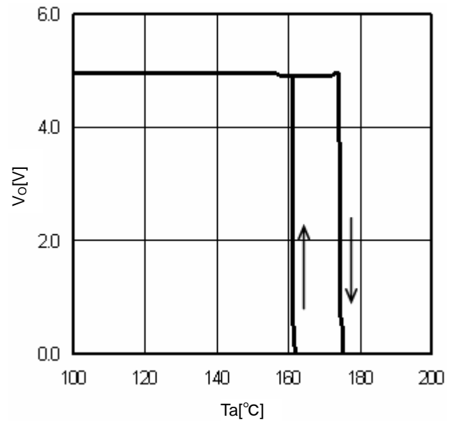
Fig.15 TSD ( I_O=0\text{mA} )
