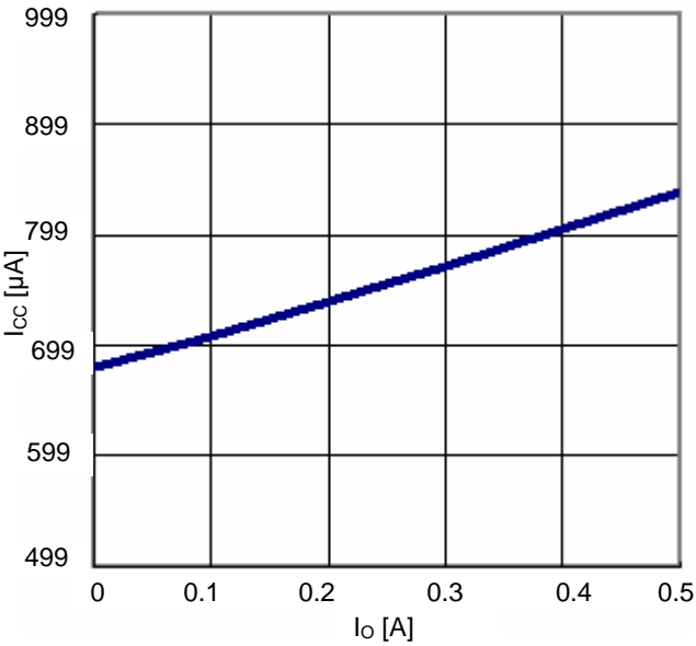
Fig.19 I_o - I_{cc}
