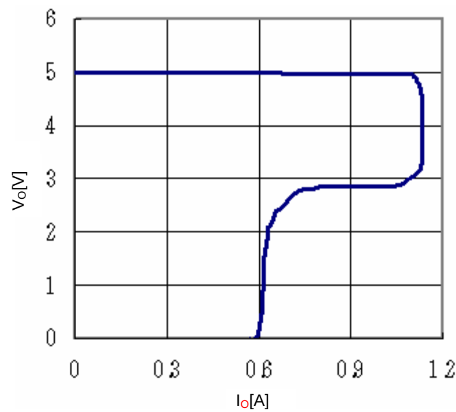
Fig.16 OCP
