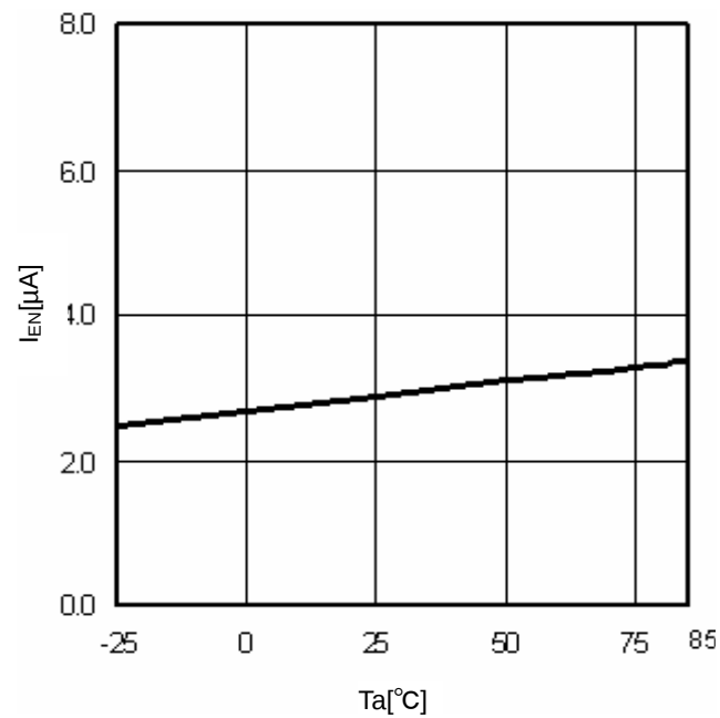
Fig.11 T_a - I_{EN}
