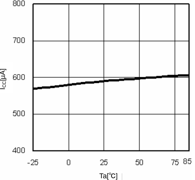
Fig.9 T_a-I_{cc}
