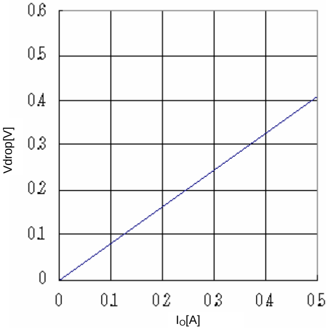
Fig.21 Minimum dropout Voltage 2 ( V_{cc}=4.5V 、 T_a=25^{\circ}C )
