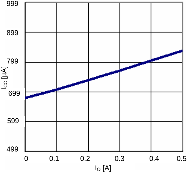
Fig.19 I_o - I_{cc}
