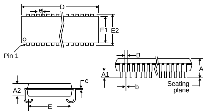
32-pin SOJ 400 mil
