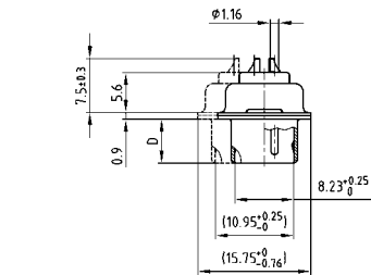
50 pos. = Dim. in ( _ )
