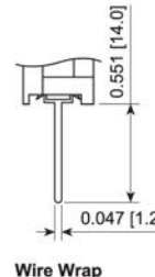
Wire Wrap
