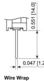
Wire Wrap
