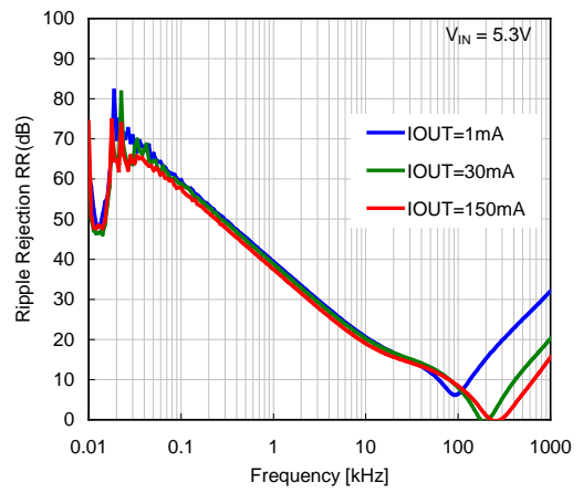
VR=3.3V
