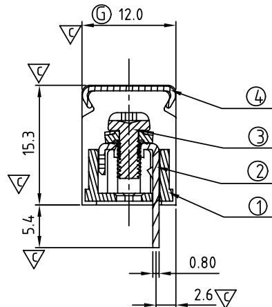
SECTION:P-P
