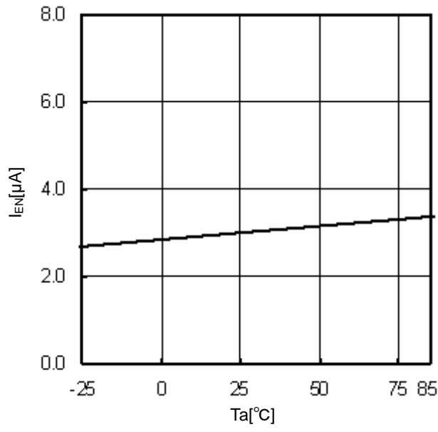
Fig.14 Ta-Ien
