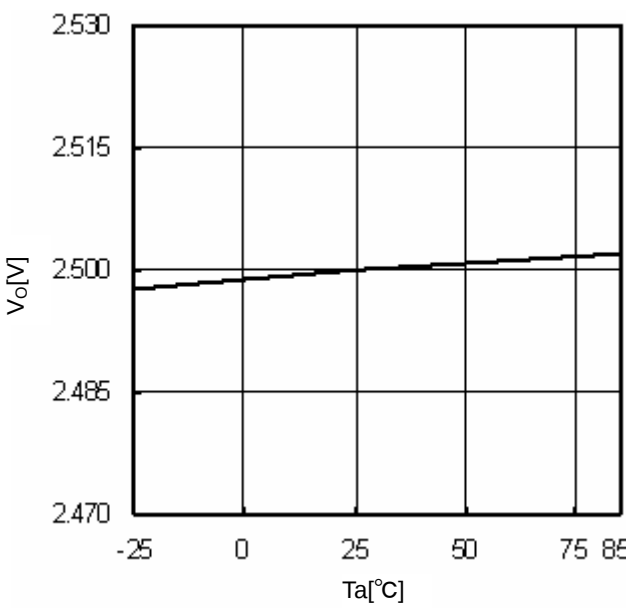
Fig.10 T_a-V_O ( I_o=0A )
