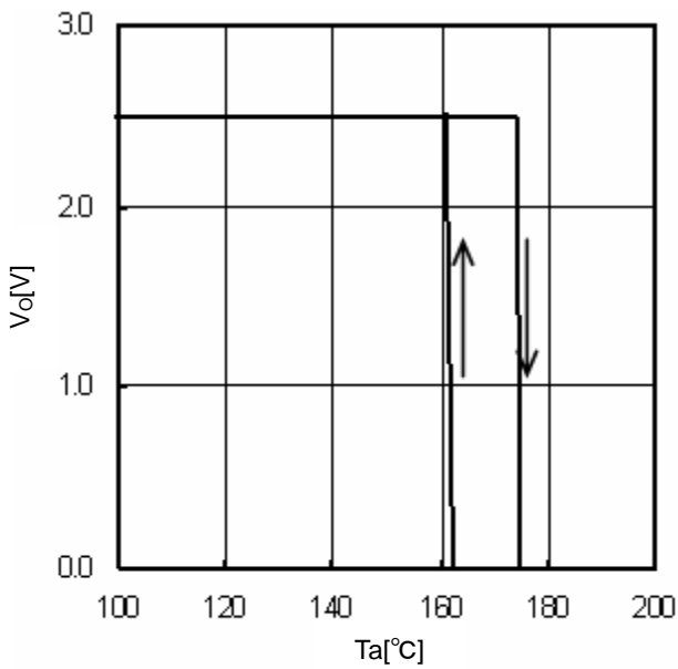
Fig.21 TSD ( I_o=0 A)
