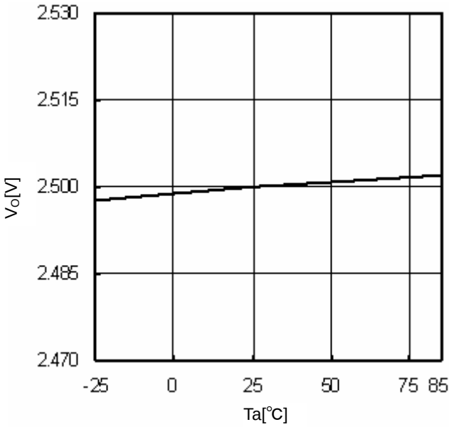
Fig.10 T_a-V_O ( I_o=0A )
