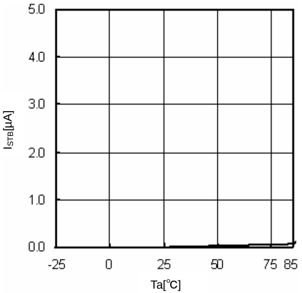
Fig.12 Ta-Istb (VEN=0V)
